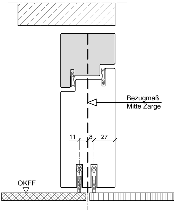
HR70-Doppelfalz 2 Bodendichtungen
