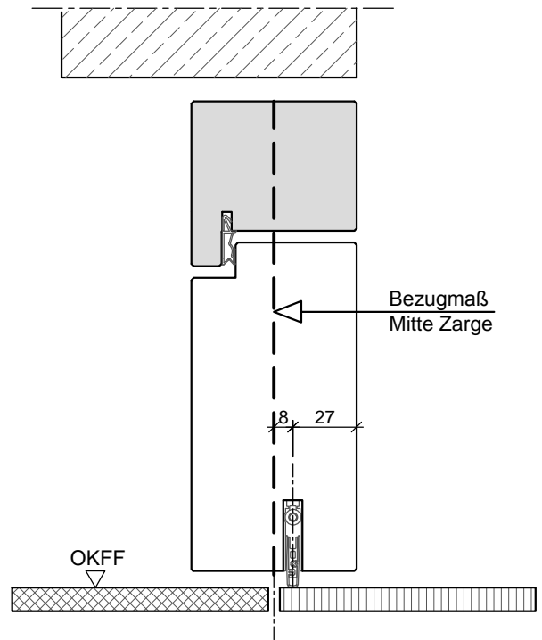
HR70-flächenbündig
