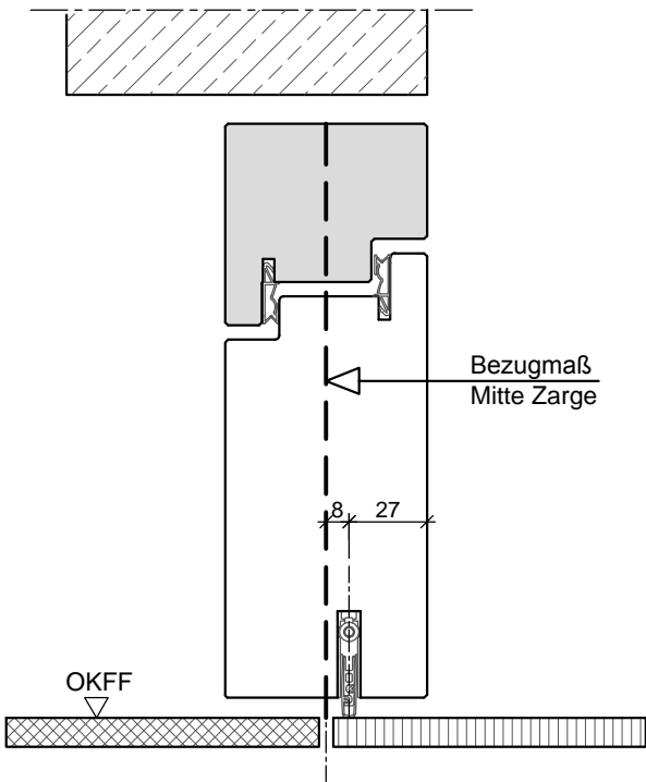
HR70-Doppelfalz
