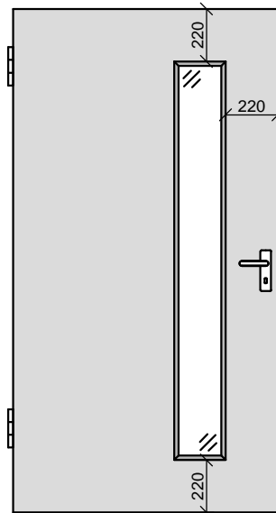
Schlitzglas
