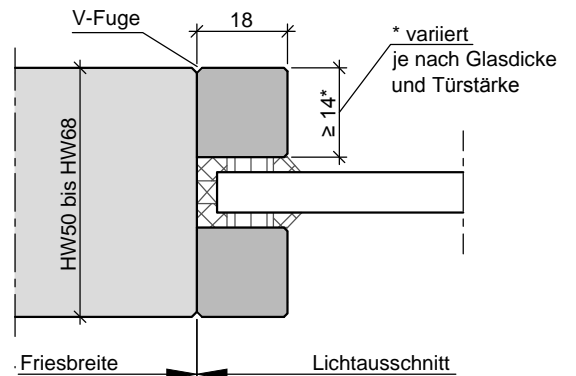
flächenbündige Glasleiste HW50 bis HW68
