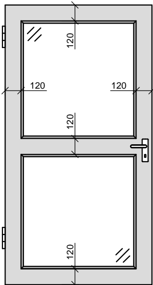
Mehrfeld Lichtausschnitt
