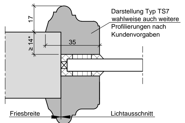
profilierte Glasleisten
