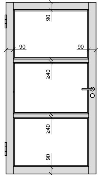
2 glasteilende Sprossen
