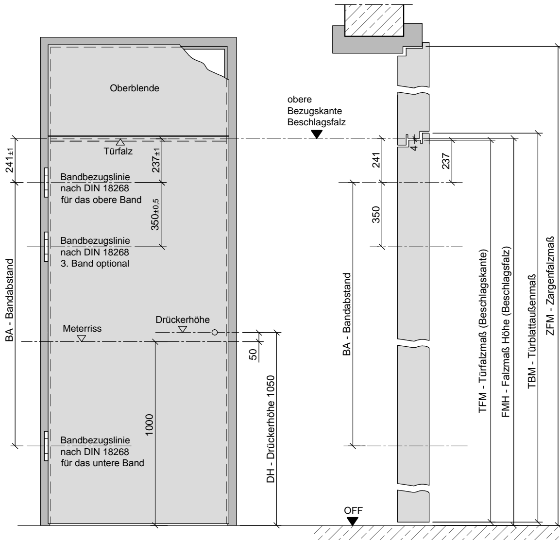
Bandbezuglinie Türblatt mit Doppelfalz mit Oberblende
