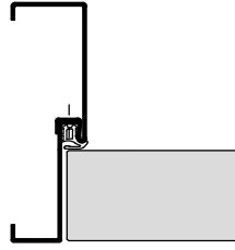
2-teilige Stahlfassungszone
