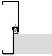
2-teilige Stahlfassungszone
