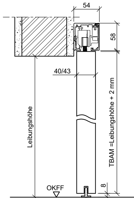
Schiebetür vor der Wand laufend ohne Durchgangsfutter Schiebetürkasten aus Aluminium
