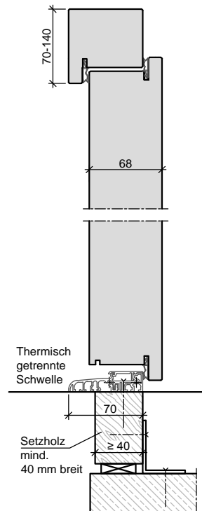
Bodenanschluss Türblatt gefälzt aufliegend
