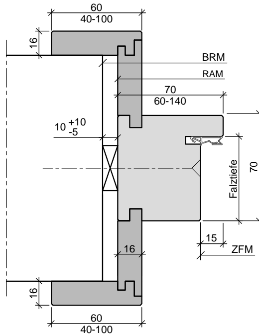
Holzstockzarge mit beidseitigem Leibungsfutter
