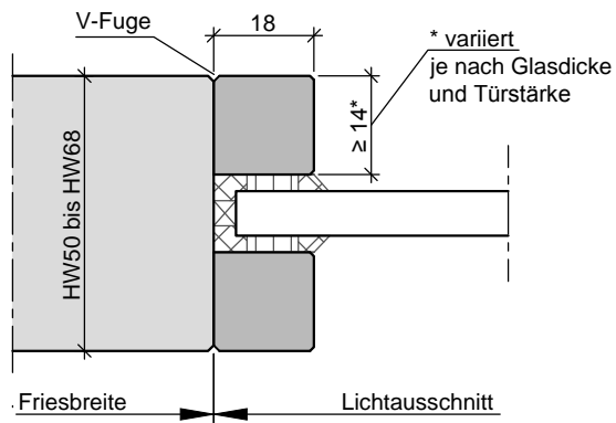
flächenbündige Glasleiste HW50 bis HW68
