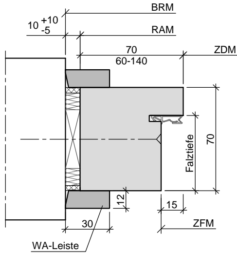
Holzstockzarge in Leibungsmontage mit Wandanschlussleisten
