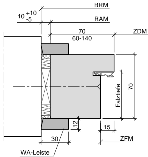
Holzstockzarge in Leibungsmontage mit Wandanschlussleisten
