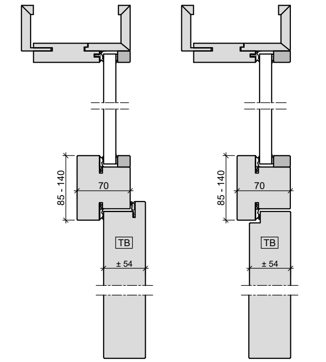
Oberlicht mit Kämpfer Türblatt gefälzt in Holzobjektzarge
