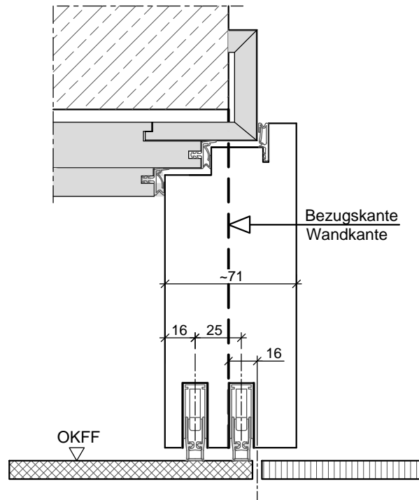
HW71-aufliegend mit Doppelfalz in Holzumfassungszarge mit 2 Bodendichtungen
