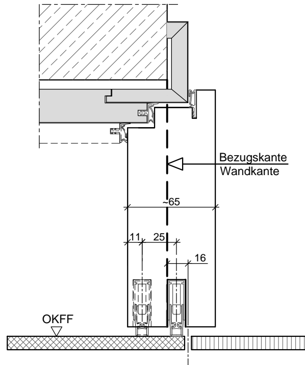
HW65-aufliegend mit Doppelfalz in Holzumfassungszarge (2. Bodendichtungen optional)
