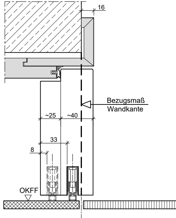
HW65-stumpf mit Leibungsfalz in Holzumfassungszarge (2. Bodendichtung optional)
