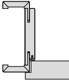
Holz-Umfassungszarge
