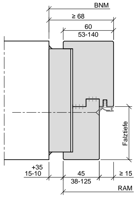
Massiv - Blockzarge mit Schattennut
