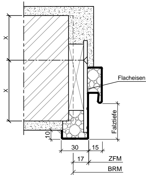
Stahlfassungszarge mit einfachem Schraubanker
