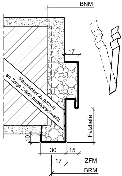
Stahleckzarge mit Mauerankerbefestigung
