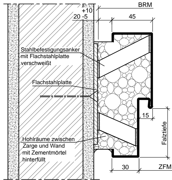
Blockzarge mit Schweißankerbefestigung in Parallelwandmontage
