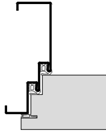
Stahl-Umfassungszarge
