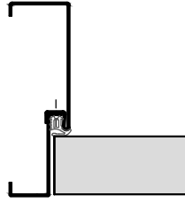
2-teilige Stahlfassungszone
