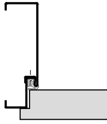
2-teilige Stahlfassungszone
