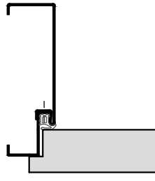
2-teilige Stahlfassungszone
