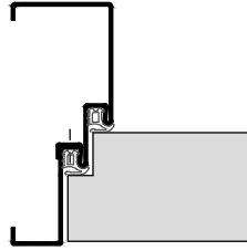
2-teilige Stahlfassungszone
