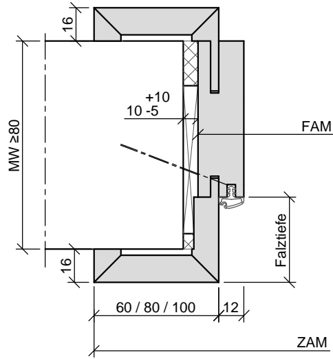
Holz - Umfassungszarge
