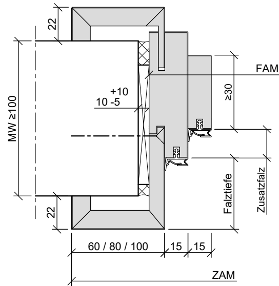
Holz - Objektzarge mit Doppelfalz
