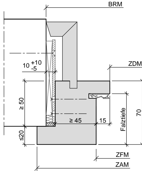
Holzstockzarge mit Ausfalzung Leibungsmontage mit Bandeisen
