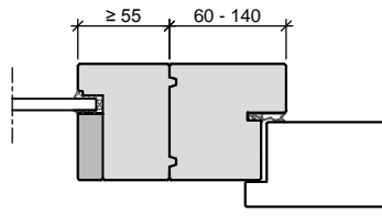
Kopplung Seitenteil / Tür Türblatt gefälzt aufliegend
