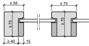
Verglasung mit glasteilender Sprosse
