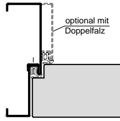
2-teilige Stahlfassungszone
