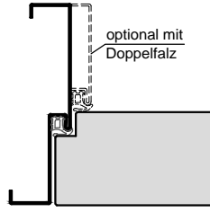
Stahl-Umfassungszarge
