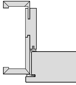
Holz-Umfassungszarge
