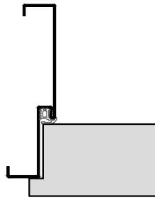
Stahl-Umfassungszarge
