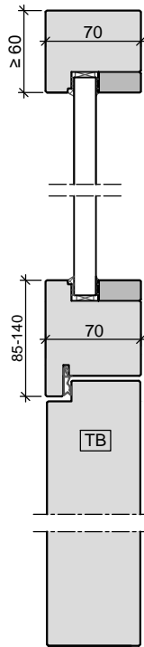
Oberlicht mit Kämpfer Türblatt stumpf in Holzstockzarge
