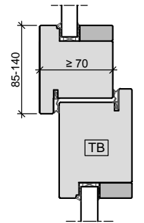
Oberlicht mit Kämpfer Türblatt gefälzt
