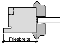
Lichtauschnitt mit profilierter Glasleiste
