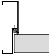
2-teilige Stahlfassungszone
