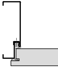
2-teilige Stahlfassungszone
