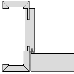
Holz-Umfassungszarge
