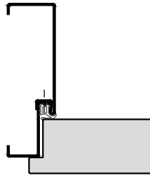
2-teilige Stahlfassungszone
